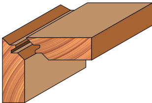
45° geringsamling
